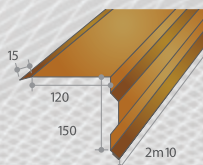
Rive 150 : 04080306
