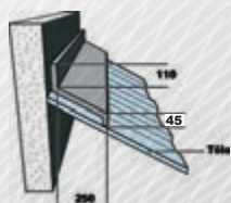
Faitière contre mur 2 m : 04080201
