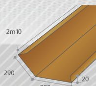
Noue en 2,10 m : 04080304
