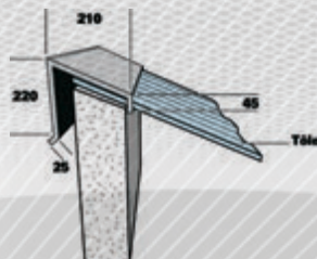
Faitière sur mur 2 m : 04080205
