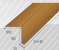
Bavette de gouttière : 04080403
