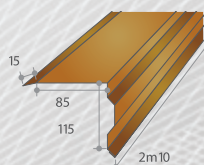
Rive 115 : 04080306
