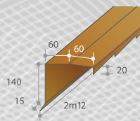
Bande de rive crantée en 2,10 m : 0408021
