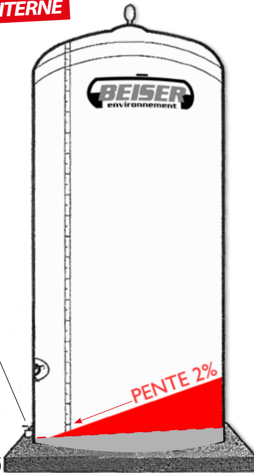
Bride de vidange avec vanne inox 316 et raccord pompier 3"
