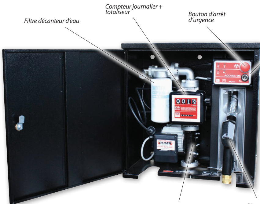
Pompe 72L/min
