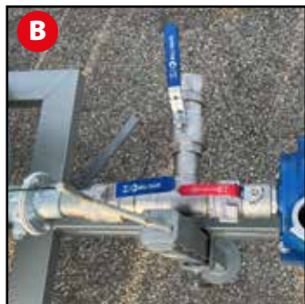
B Kit complet pour aspiration et remplissage (complément pour la pompe à cardan) Réf. 01990700131
