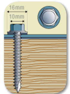
Vis pour charpentes bois
