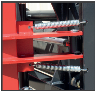
Ouverture flottante des pinces avec stabilisation par ressorts
