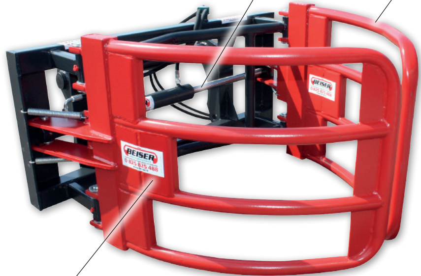
Vérin centrale double effet
