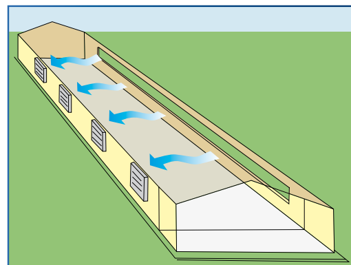
Exemple d'installation
