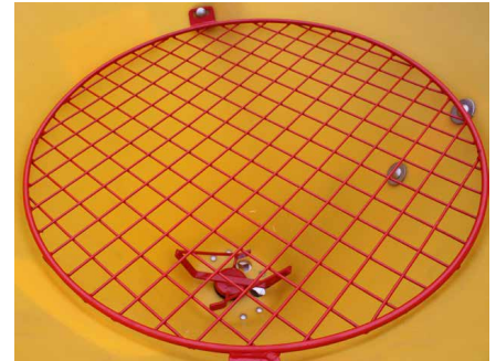
> Grille de protection et agitateur articulé
